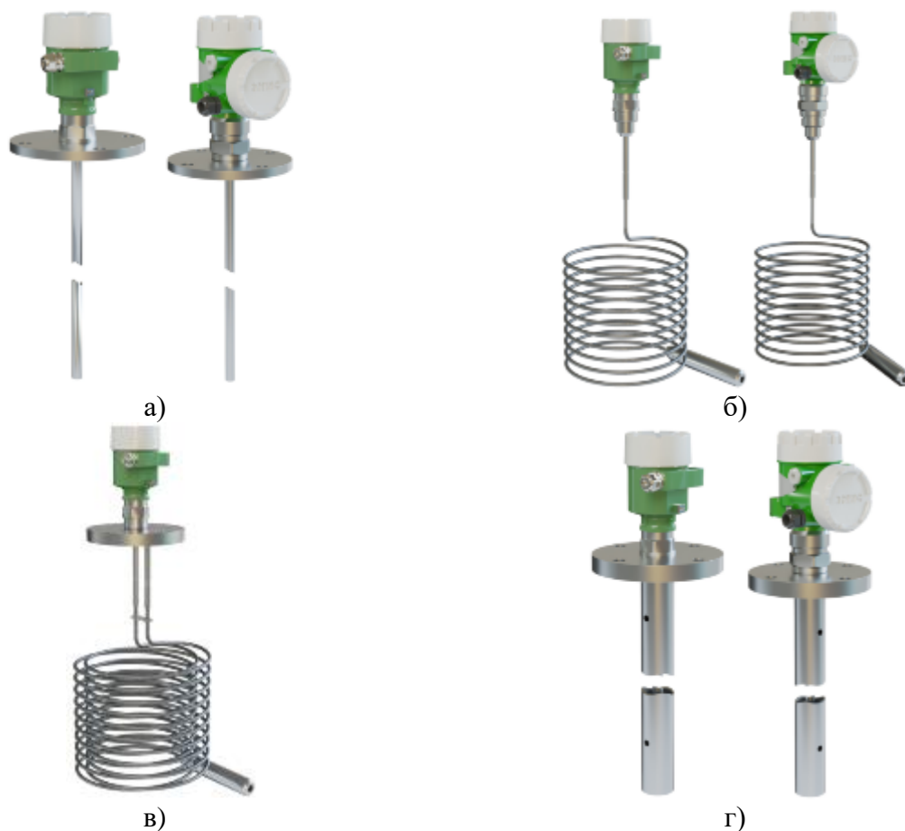
а) со стержневым зондом; б) с тросовым зондом; в) с двойным тросовым зондом; г) с коаксиальной трубкой;
